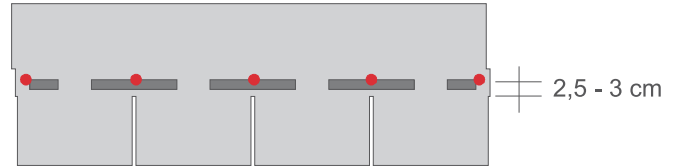
▲ Drawing Nr. 5
